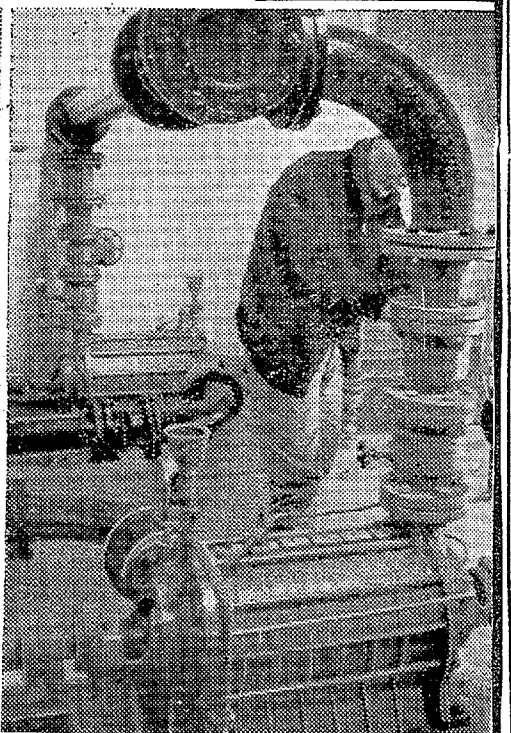
20馬力の揚水ポンプを二基備えたポンプ室 自家発電設備もあり停電でも断水しない
