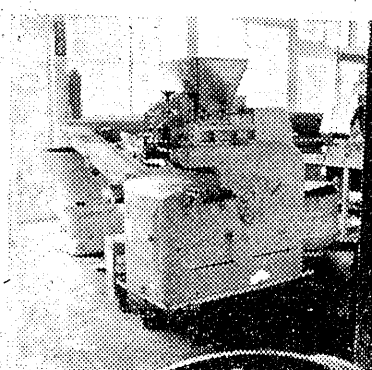
デバイダー (分割機) 毎時 3000コ
