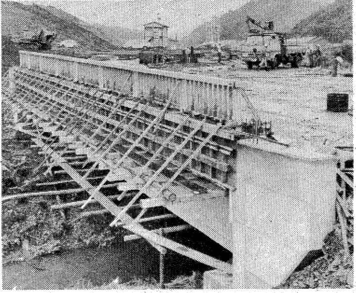
取り付け道路入り口の架橋工事
